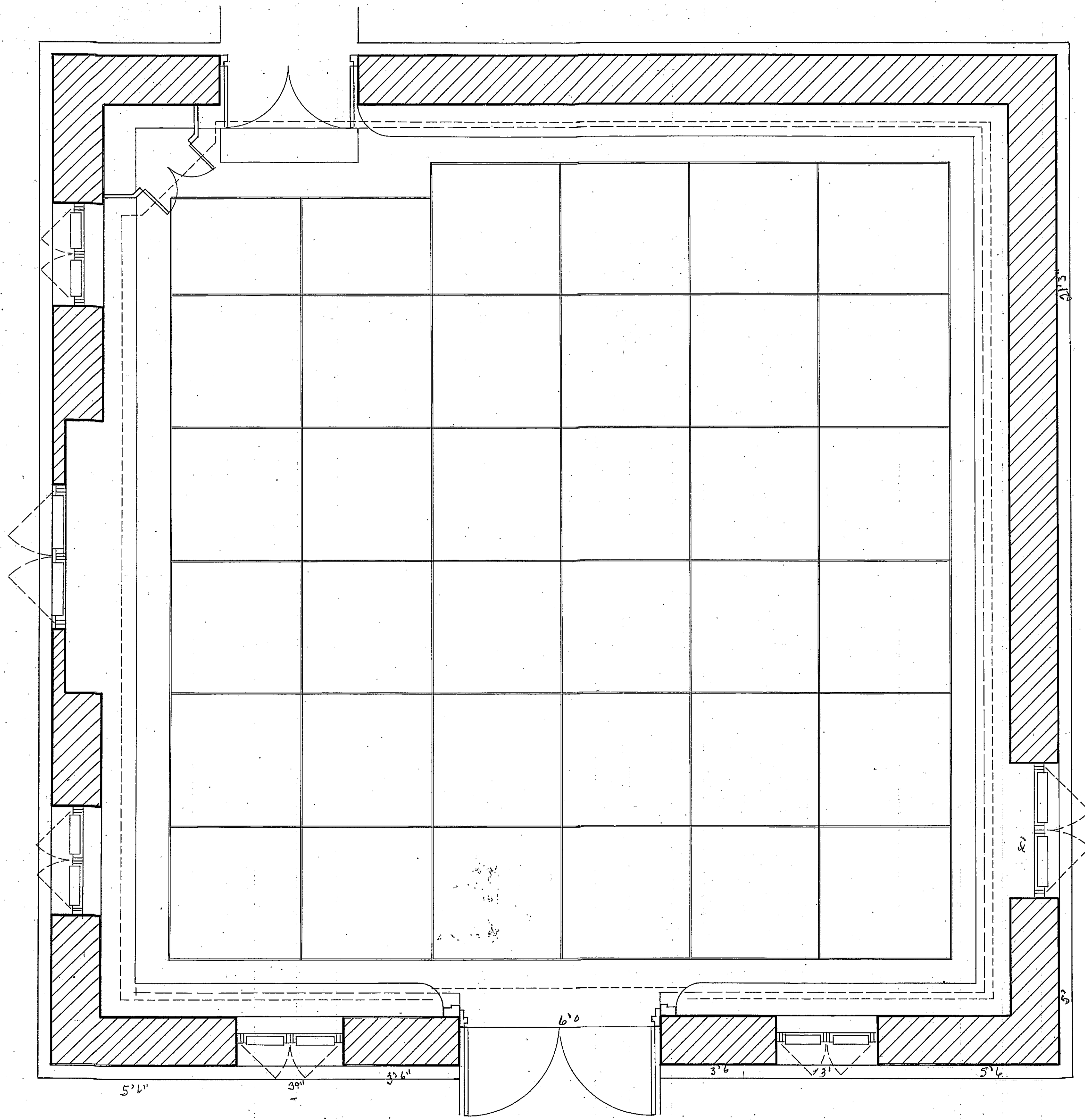
PLANTA Y PATRON DE PISO
