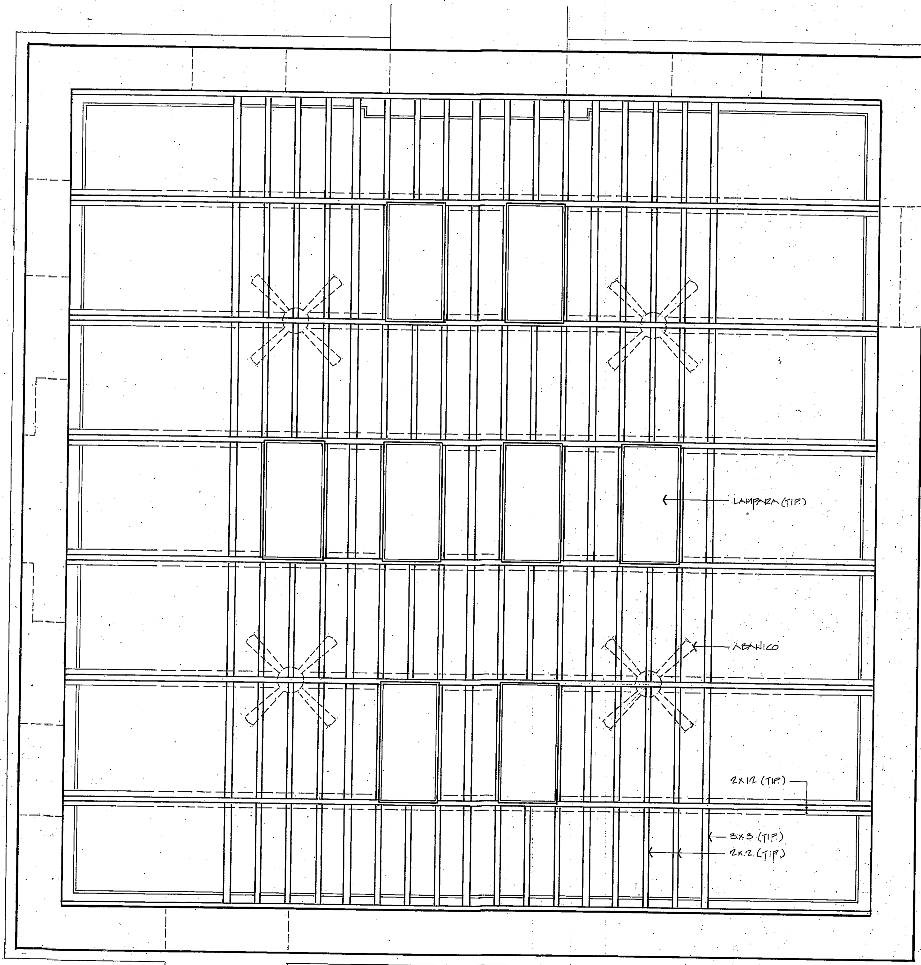
PLANTA DEL "TRELLIS" REFLEJADO 1/2" = 1'-0"
