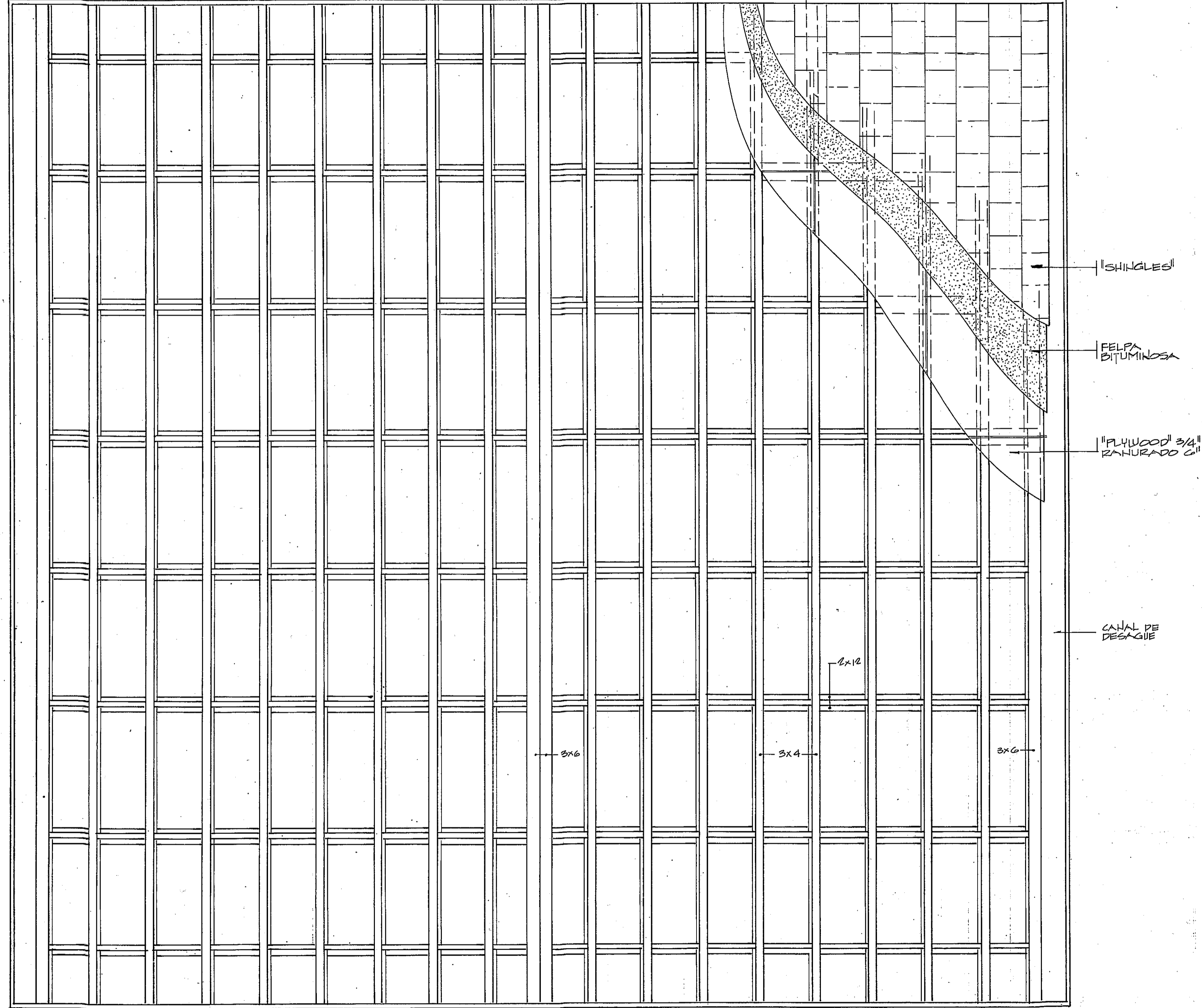
PLANTA DEL ENTRAMADO DE TECHO 1/2" = 1'-0"
