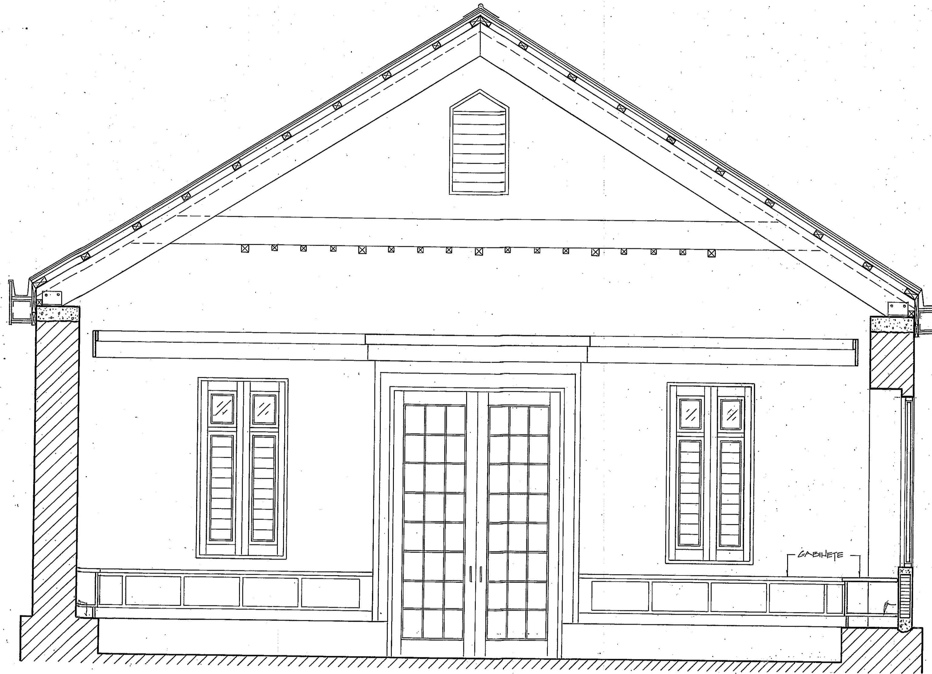
SECCION TRANSVERSAL
