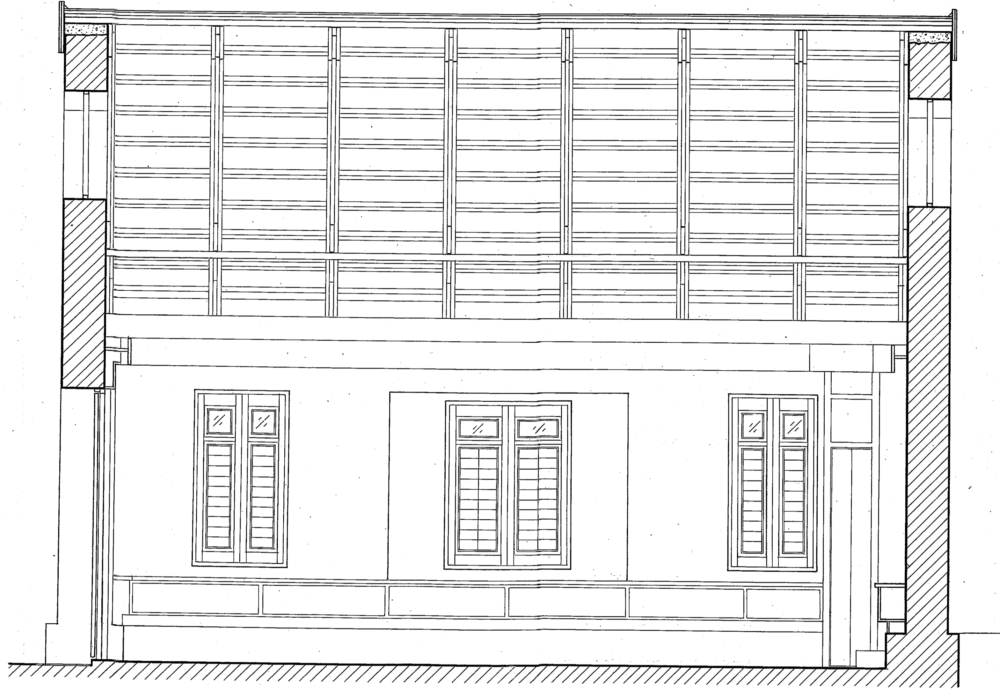
SECCION LONGITUDINAL 1/2" = 1'-0"
