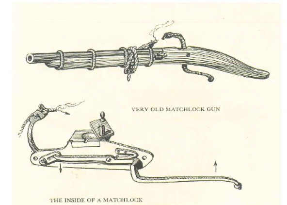
เครื่องลั่นไกจุดชนวนของปืนคาบซุด (ที่มา : http://blindkat.hegewisch.net/pirates/matchlock.jpg )
